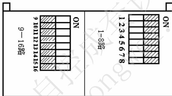
16 路输入板外形图
