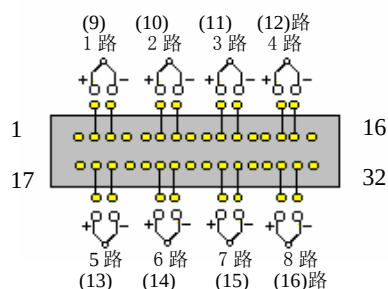
热电偶信号输入接线图:
